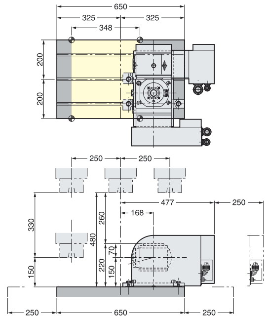
5AX-DD200
